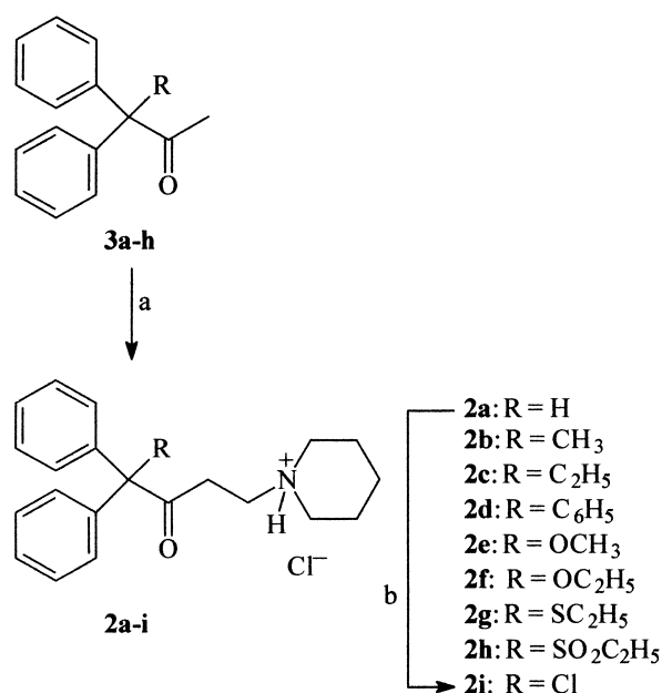
Scheme 1. (a) CH 2 O, piperidine hydrochloride, HCl, CH 3 OCH 2 –CH 2 OH, reflux, (b) Cl 2 , THF, rt.
